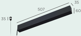
base B50
