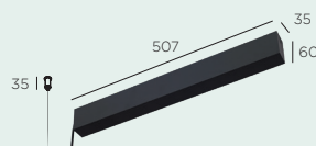
base B50
