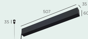
base B50
